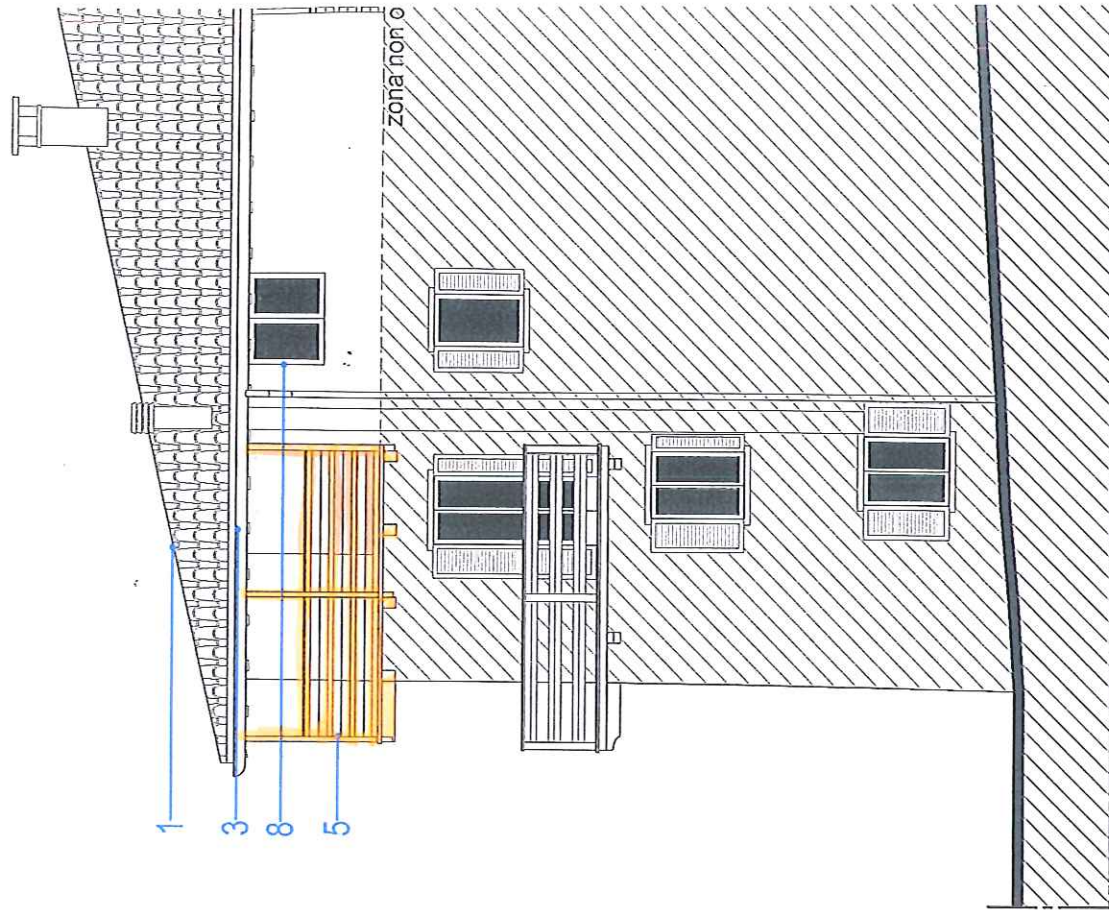
PROSPETTO EST
