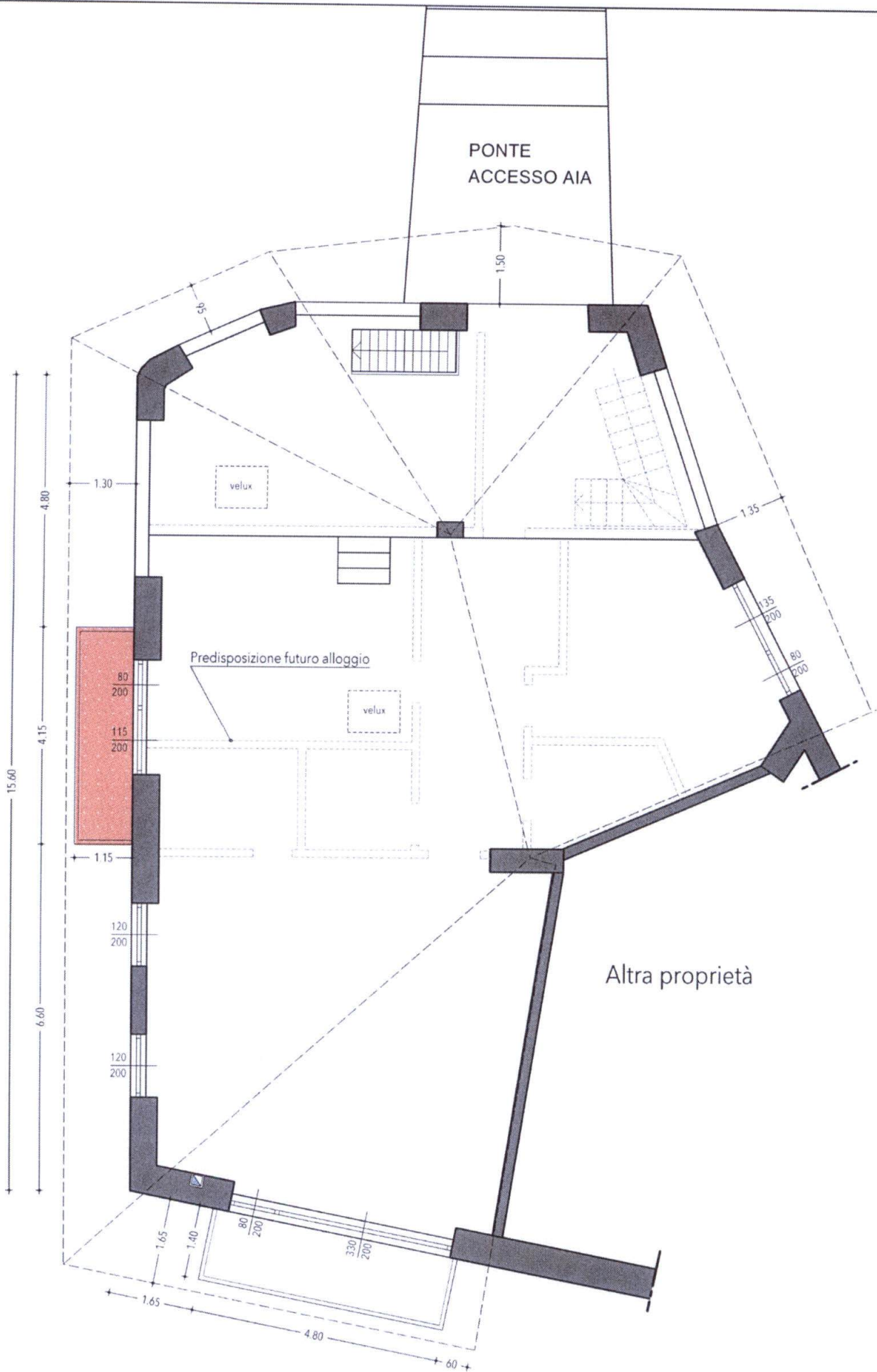
Piano sottotetto 1:100
